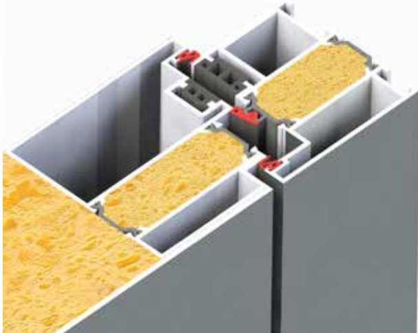
Flächenbündiges Türblatt aus Aluminiumblech
