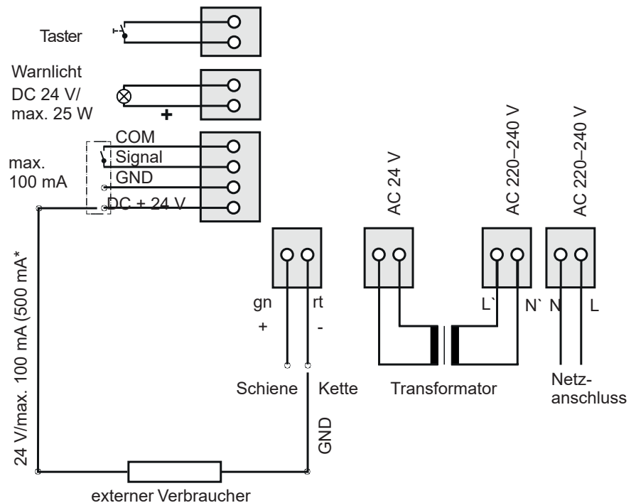
Abb. Anschlussplan Wandsteuerung
