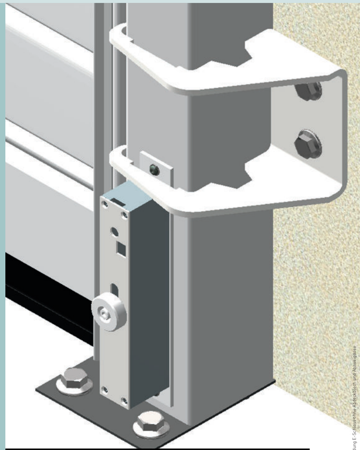
Integriertes E-Schloss mit zusätzlichem Verstärkungsprofil**
