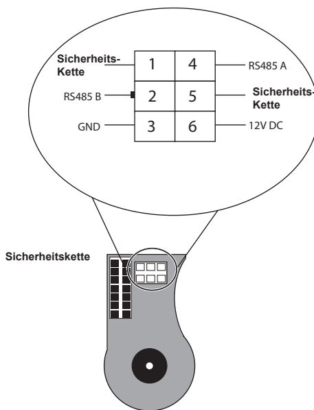
Absolutwertgeber (Encoder)
