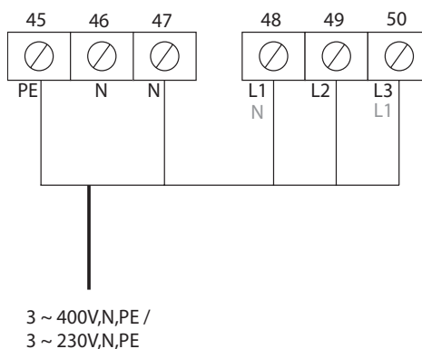
Netzanschluss
